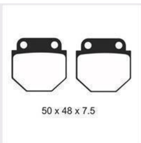
PASTILLA10** JGO PASTILLA FRENO CUSTOM GIL YL125 /HJ125/ EN 125/GN 125
