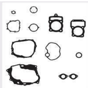
JUNTA22** JGO JUNTA MOTOR ZANELLA ZTT 200 SIN BALANCEADOR (VARILLERA) 63.5MM
