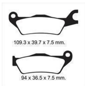
PASTILLA18** JGO PASTILLA FRENO HONDA INVICTA 150 / GIXXER 150
