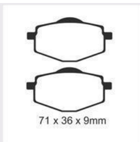
PASTILLA9** JGO PASTILLA FRENO YAMAHA YBR 125 CHINA
