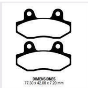
PASTILLA3** JGO PASTILLA FRENO GILERA SMASH (S/MUECA)
